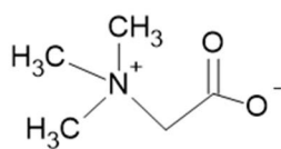
Betaine (Be)
