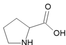
Proline (Pro)
