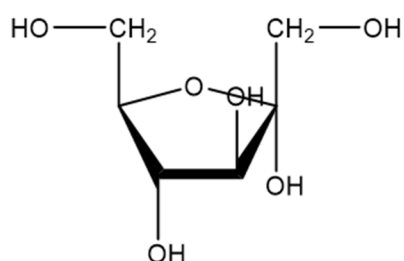
Fructose (F)
