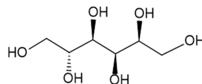
Sorbitol (So)
