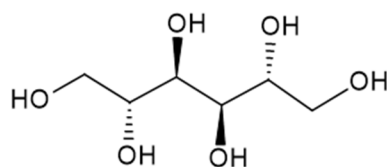
Mannitol (Mo)
