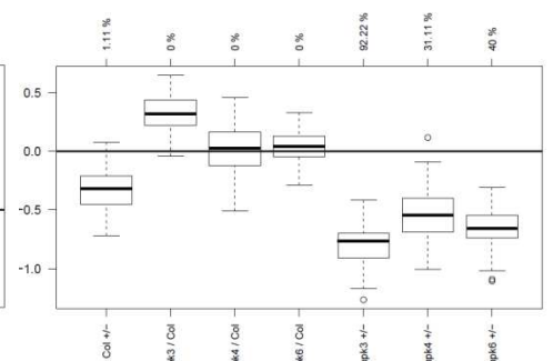
Cluster 24 / 91 genes
