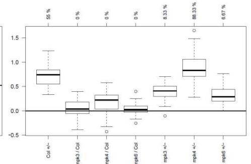
Cluster 15 / 58 genes
