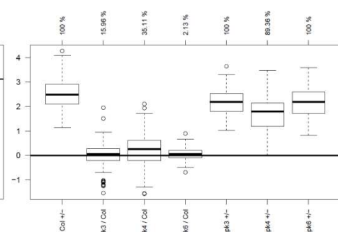
Cluster 20 / 92 genes
